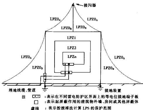
图 3.2.2 建筑物雷电防护区 (LPZ) 划分
